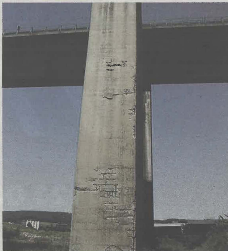
Una de las pilastras del viaducto de Somonte, en mal estado. | LNE
